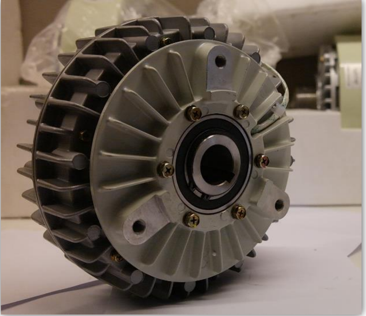
Şekil 1. UTF-D serisi manyetik tozlu fren.
